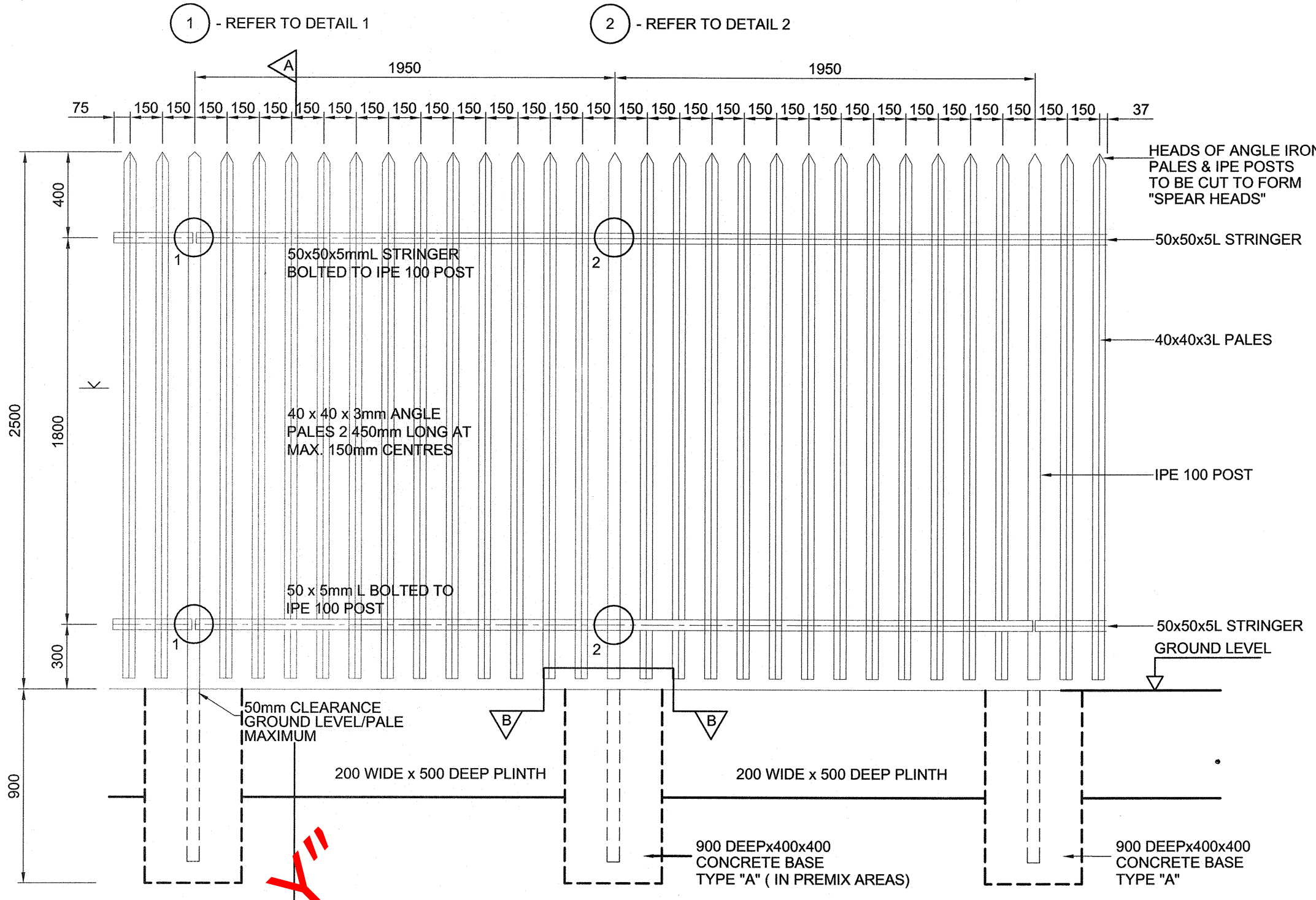
ELEVATION 1:20
